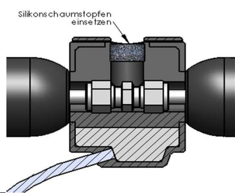
T-Stück NW4
